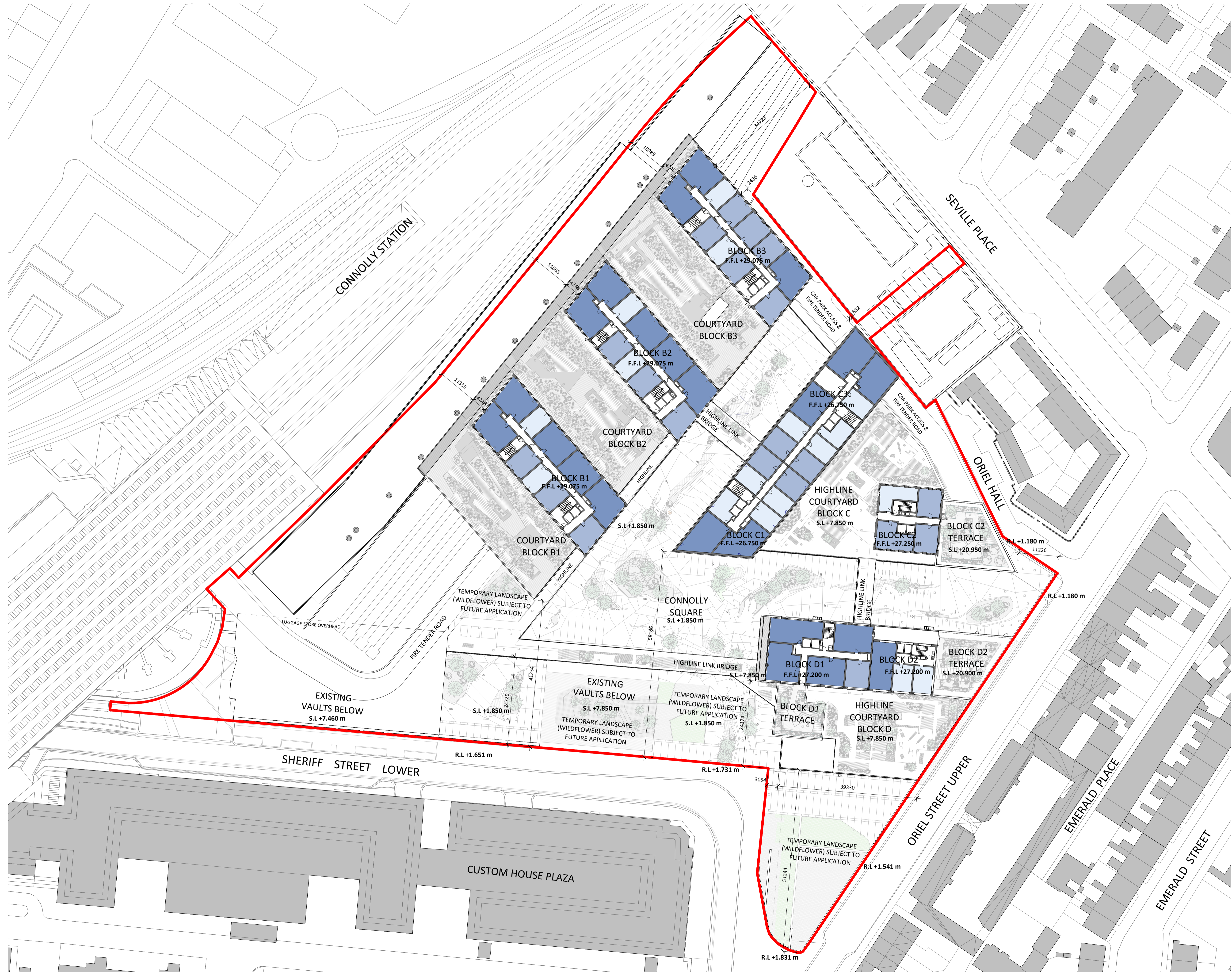
1 SITE LAYOUT PLAN - LEVEL 07 1 : 500
